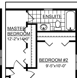
OPTIONAL ENSUITE PLAN 5015-0010
